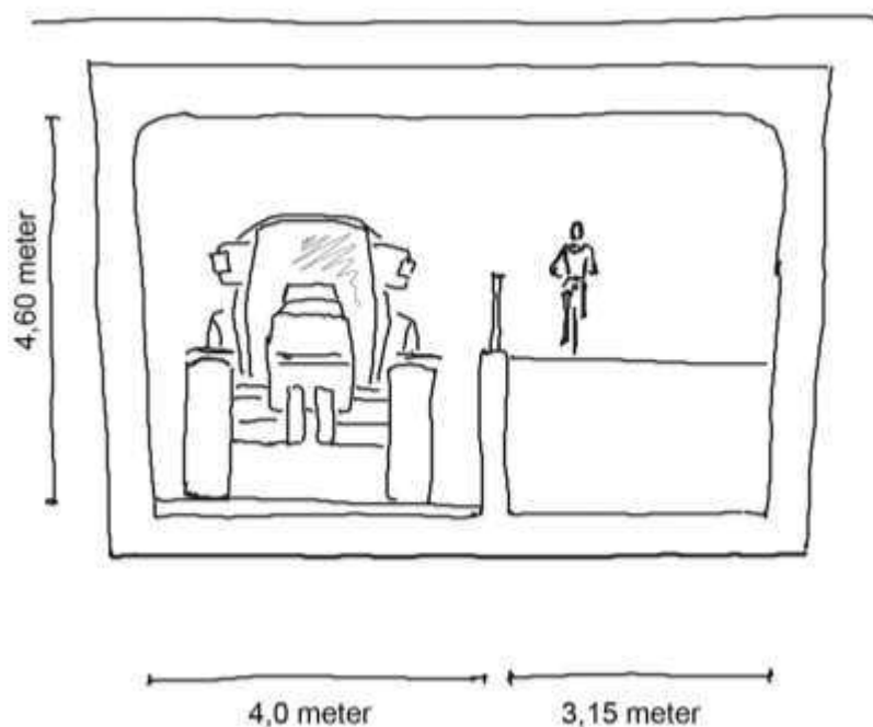
Figuur 4.6 principeprofiel voor de tunnel
